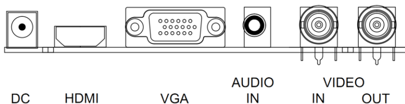
Рис. 1 Разъемы на задней панели
